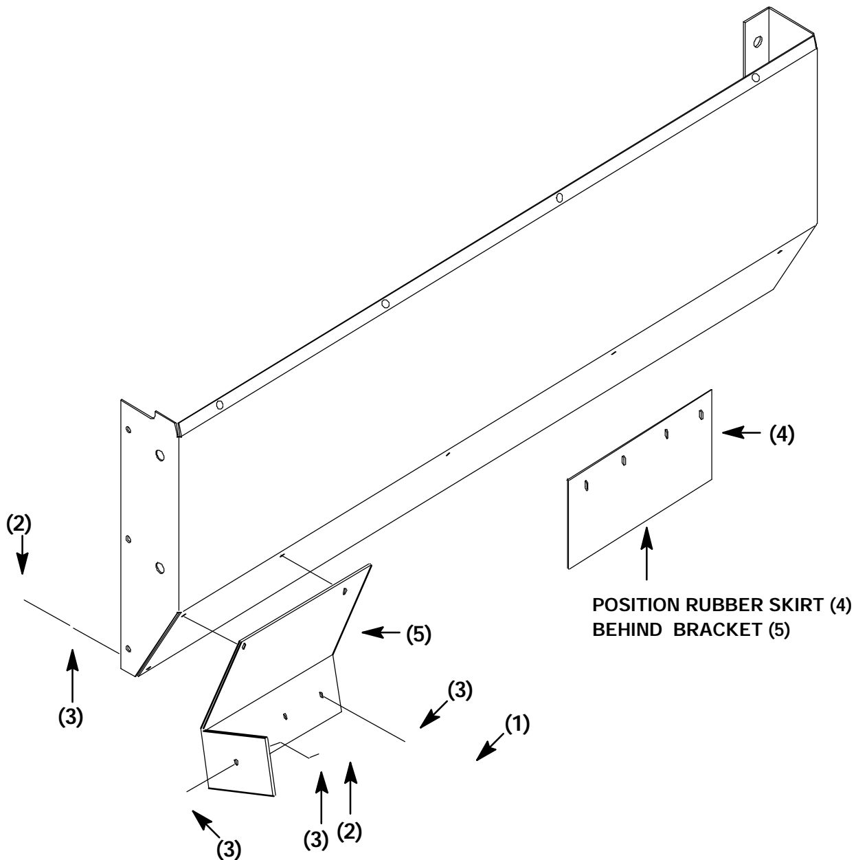
FIG. 3 - LH Brush Door Assembly
