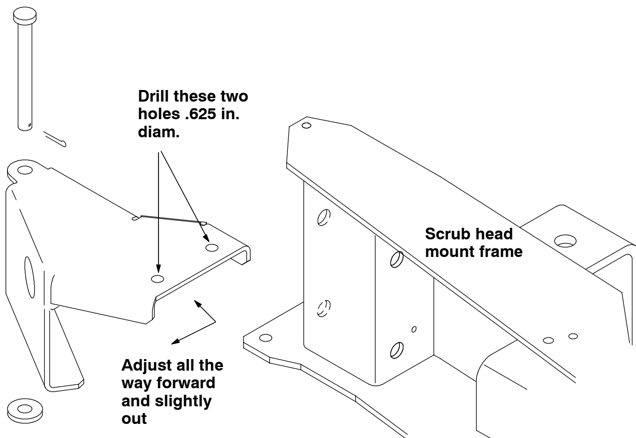
FIG. 4 - OPTIONAL SE SIDE SQUEEGEE GUARD
